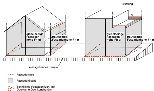
Messweisen der Fassadenhöhen bei Sattel- und Attikadach
