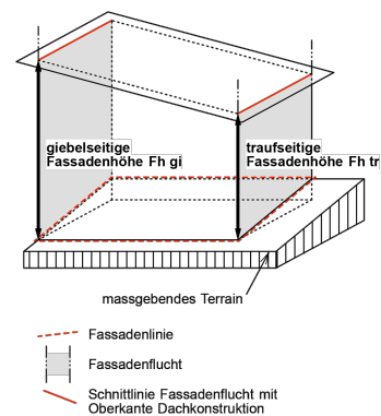
Messweise der Fassadenhöhe bei einem Pultdach
