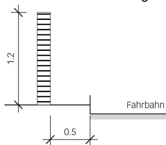
Fahrbahn ohne Gehweg
